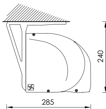
Montaggio a soffitto Ceiling installation
