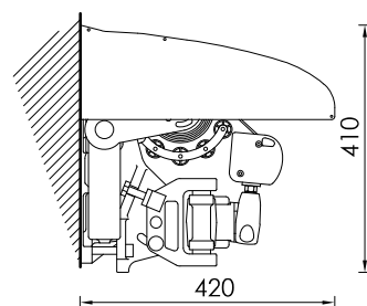
Montaggio con tettuccio Installation with a hood
