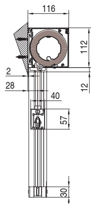
QUADRO - SQUARE A-A
