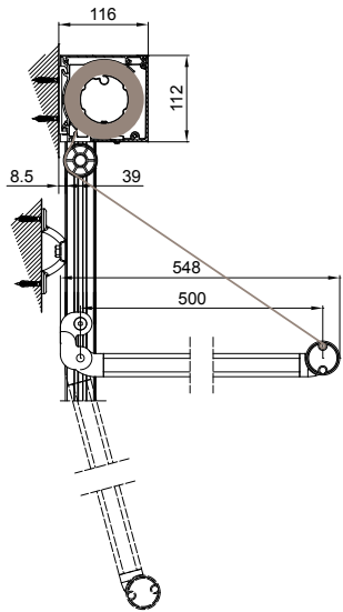
QUADRO - SQUARE A-A
