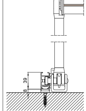
guida a parete - wall guide B-B
