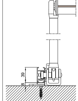
guida a nicchia - niche guide B-B
