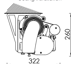
Montaggio a soffitto Ceiling installation
