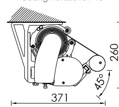
Montaggio a soffitto 45° Ceiling installation 45°
