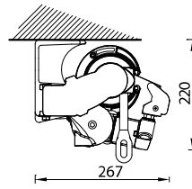
Installazione a soffitto Ceiling installation
