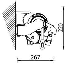
Installazione a parete Wall installation
