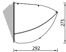
Installazione con tettuccio Installation with hood
